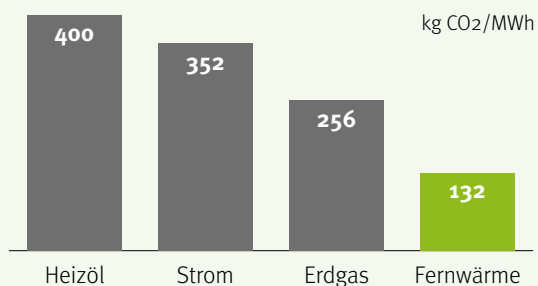
CO 2 -Emission unterschiedlicher Heizungen je MWh Nutzenergie
