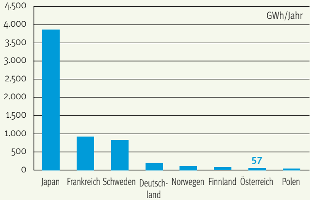
Fernkälteproduktion im internationalen Vergleich (2010/2011)
